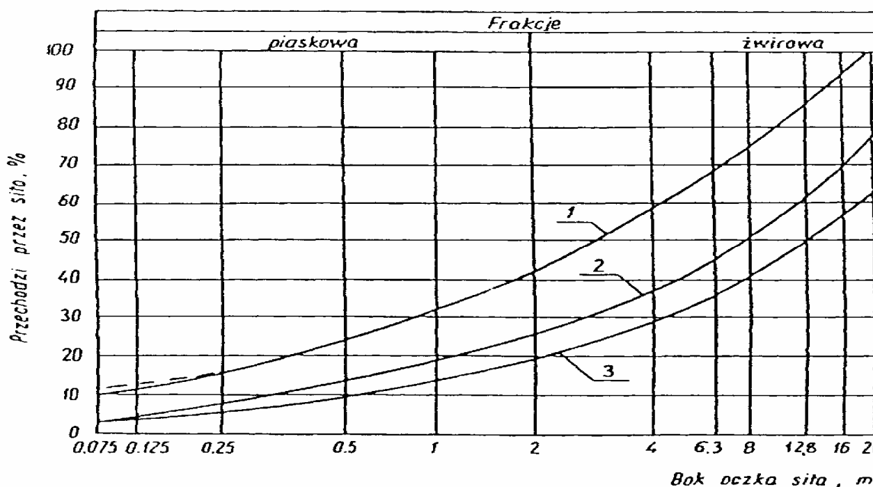
Rys. 1 Krzywa uziarnienia kruszywa na wykonanie podbudów stabilizowanych mechanicznie.
